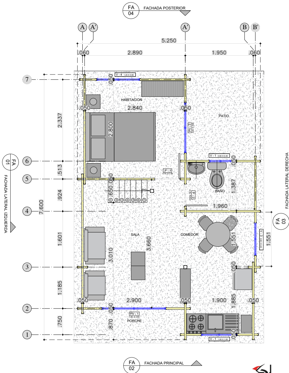
PLANTA BAJA TINY HOUSE 39 M2
