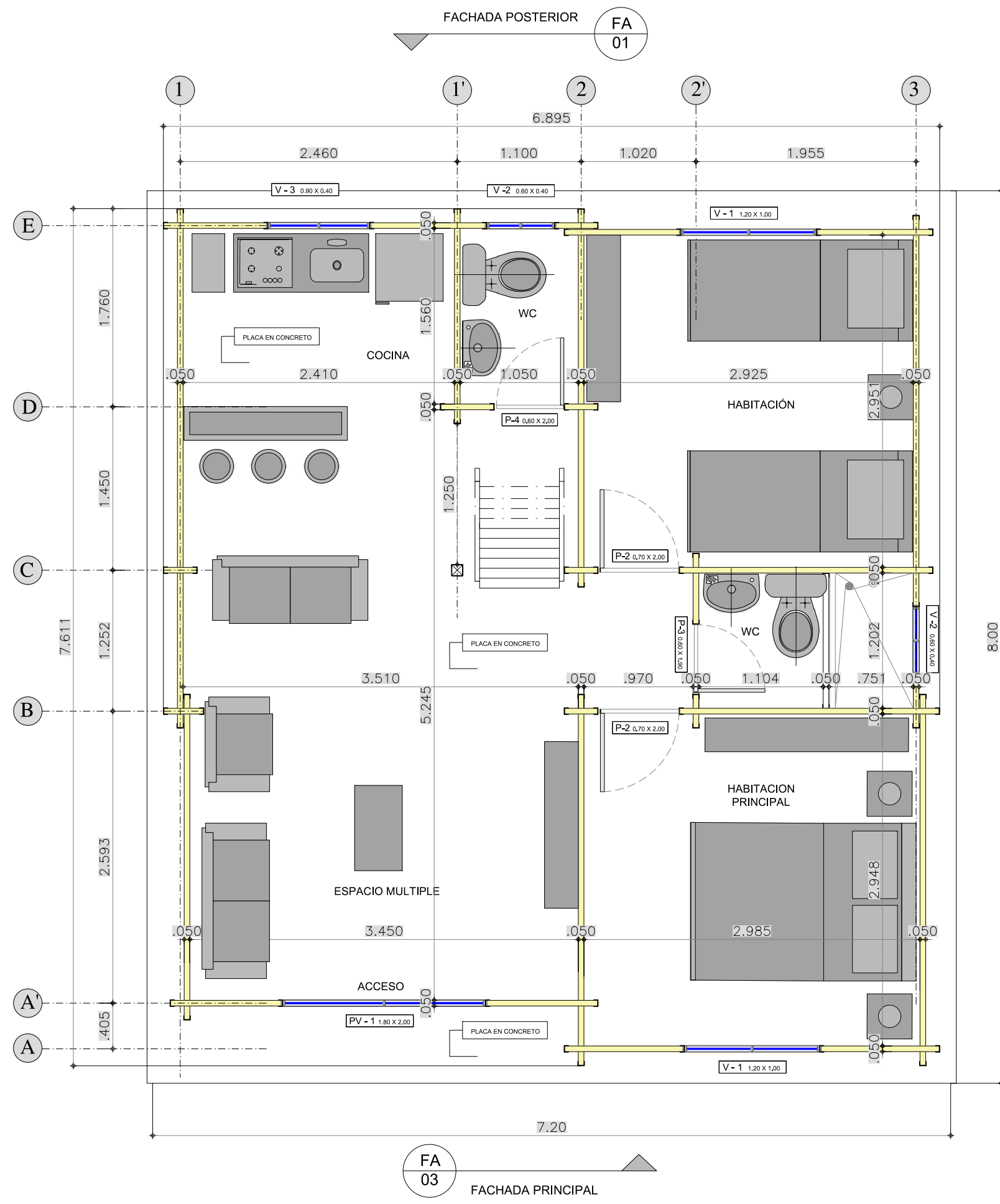
PLANTA PRIMER PISO
