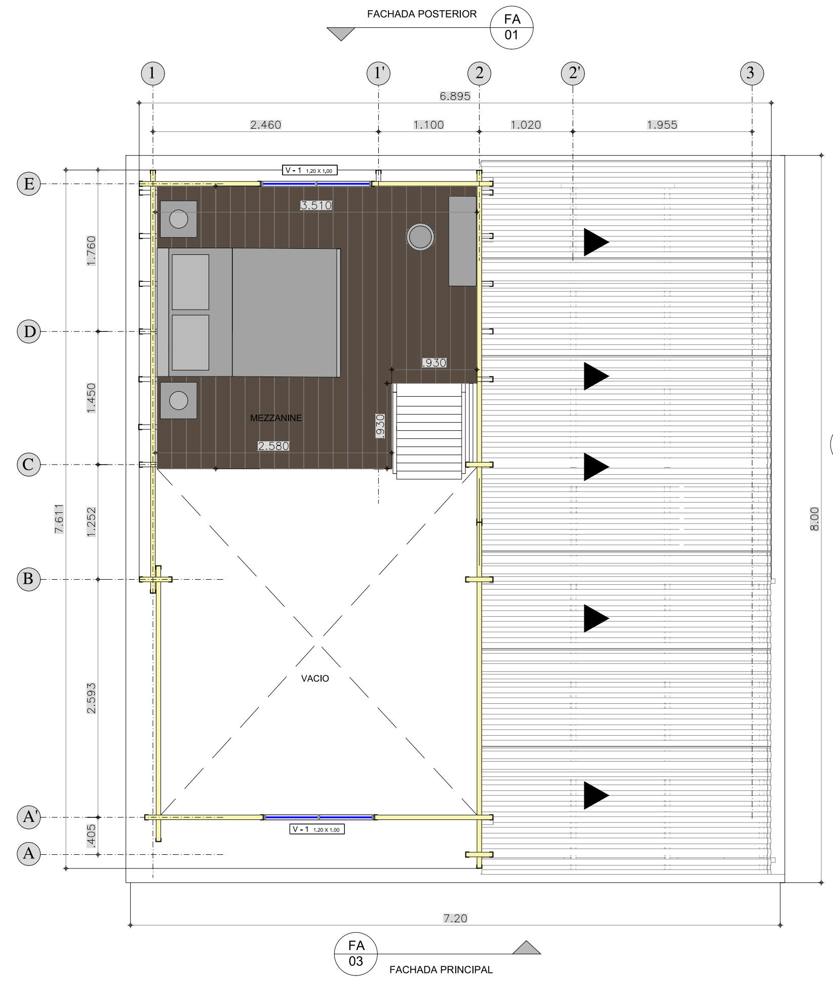
PLANTA MEZZANINE CASA
