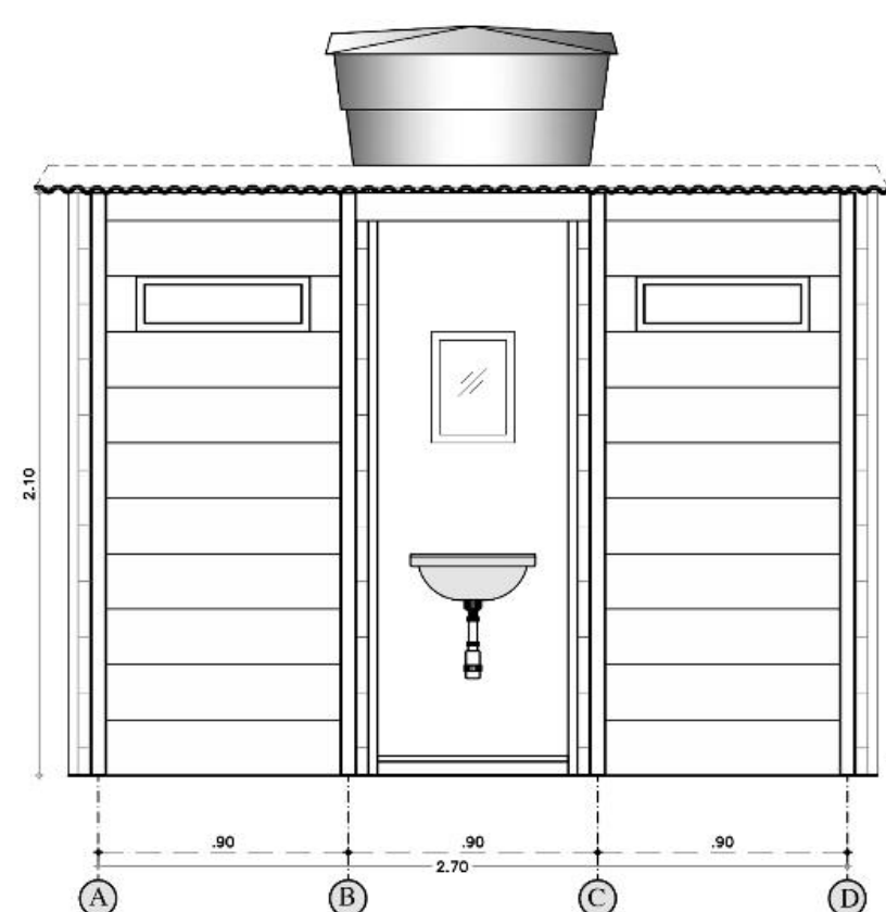
FACHADA PRINCIPAL ESC : 1:25
