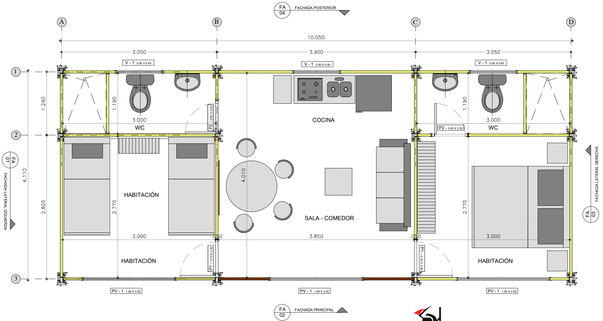
PLANTA ARQUITECTONICA CASA KIT 41 M2
