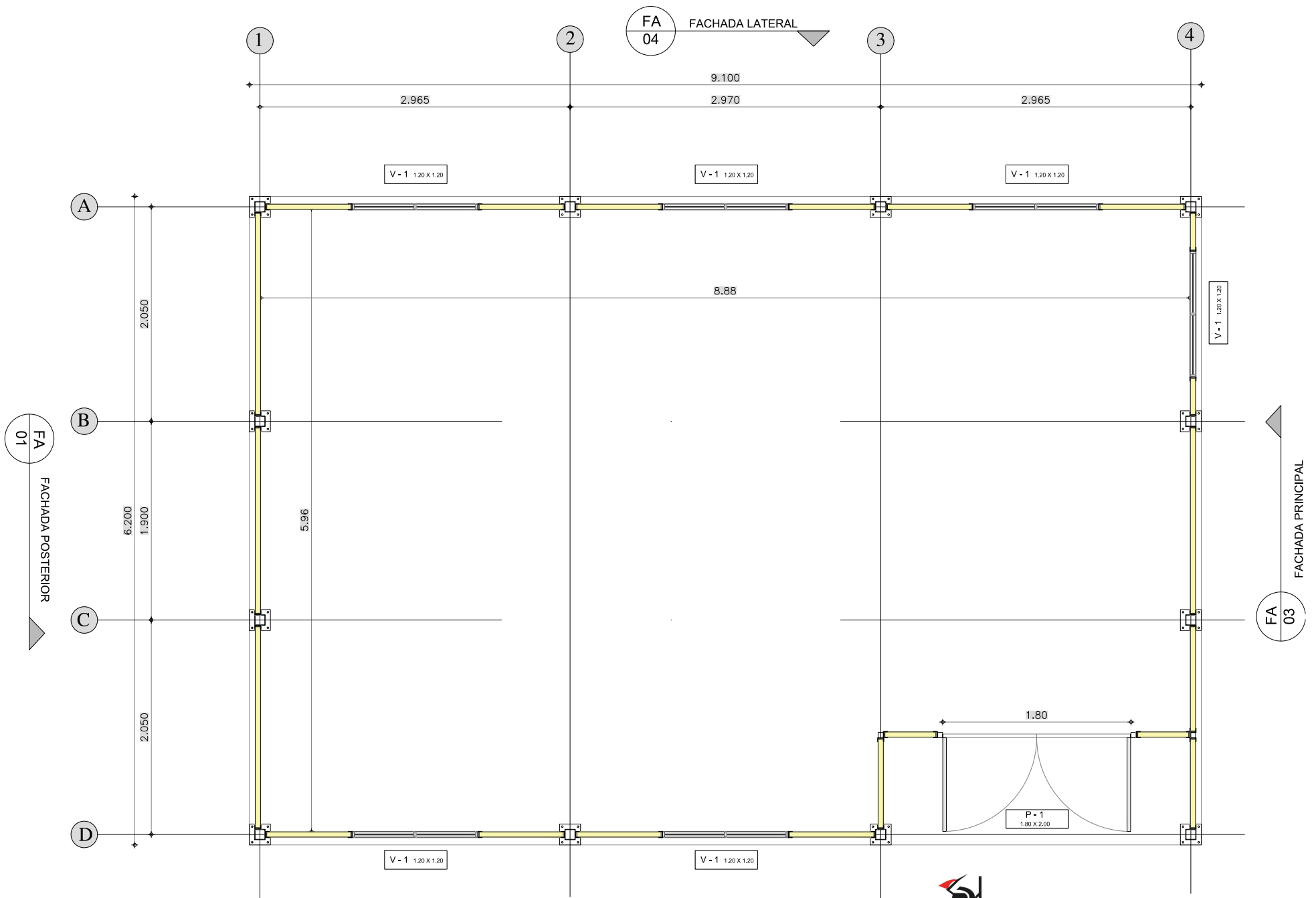
PLANTA GENERAL ARQUITECTONICA AULA KIT 54 M2
